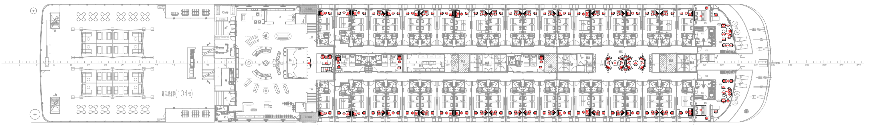
甲板标高: 40m, 豪华大桌: 4m, 餐椅间距: 2m, 内舱间距: 3m (走道按实际, 走道扶手, 带灯脚)
